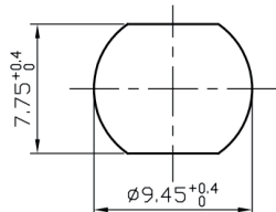
Hullbilde for DD-hull
