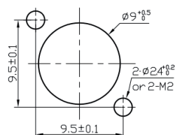
Hullbilde for oval og firkantet flens
