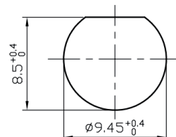
Hullbilde for D-hull
